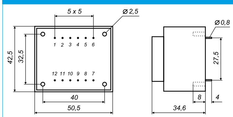
Dimenzije v mm - Pogled s strani priključkov
