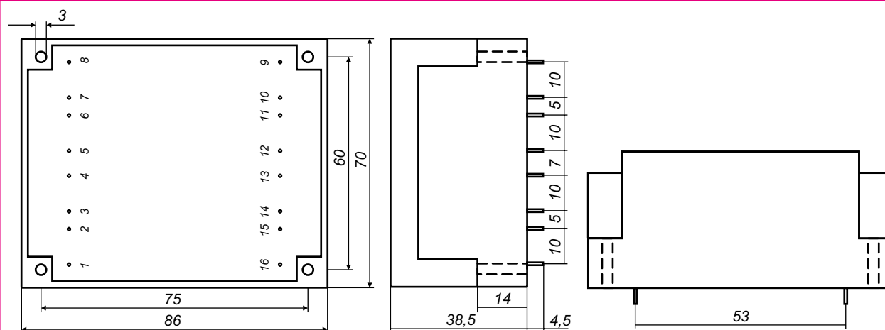
Dimenzije v mm - Pogled s strani priključkov
