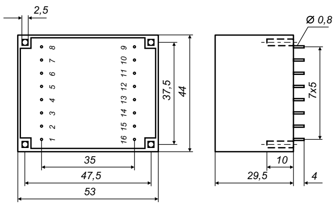
Dimenzije v mm - Pogled s strani priključkov
