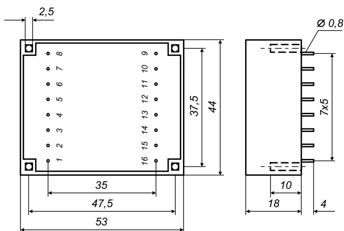
Dimenzije v mm - Pogled s strani priključkov
