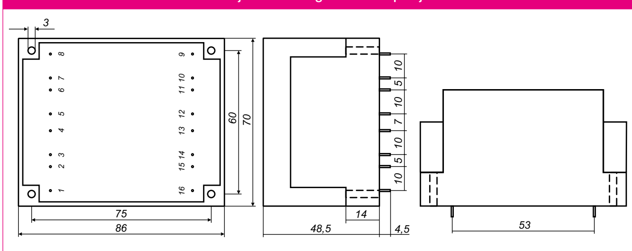
Dimenzije v mm - Pogled s strani priključkov
