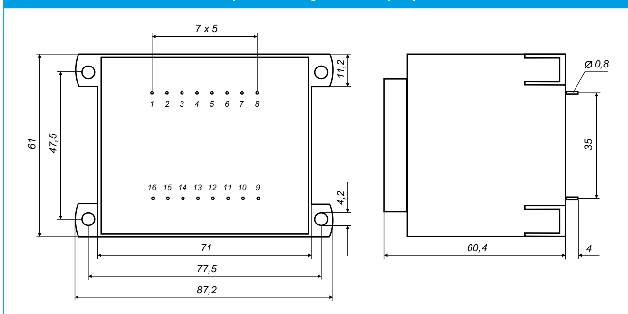
Dimenzije v mm - Pogled s strani priključkov
