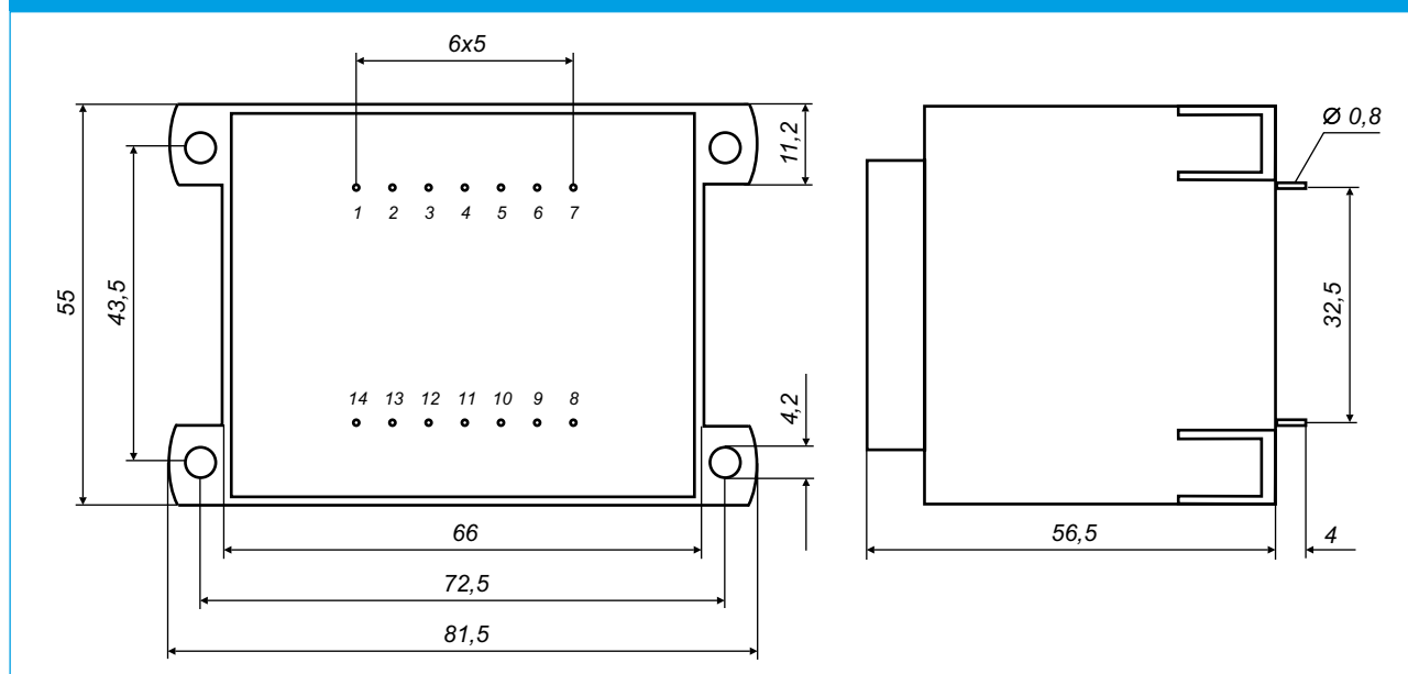
Dimenzije v mm - Pogled s strani priključkov
