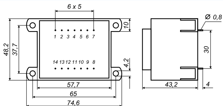
Dimenzije v mm - Pogled s strani priključkov
